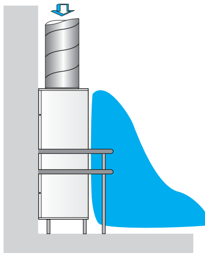
LSH anslutning ovanifrån, montage på vägg. Benstativ SBH (tillbehör) samt påkörningsskydd SPH (tillbehör).
