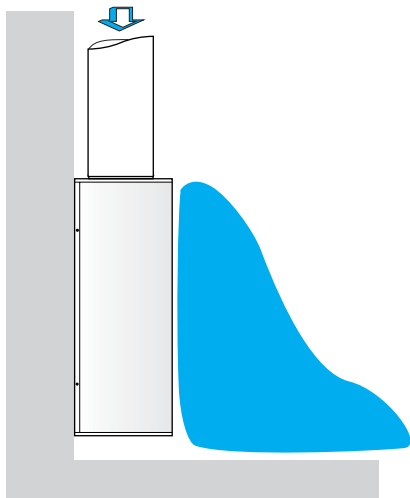
LSH anslutning ovanifrån, montage på vägg. Längsfalsad anslutningskanal CK (tillbehör).
