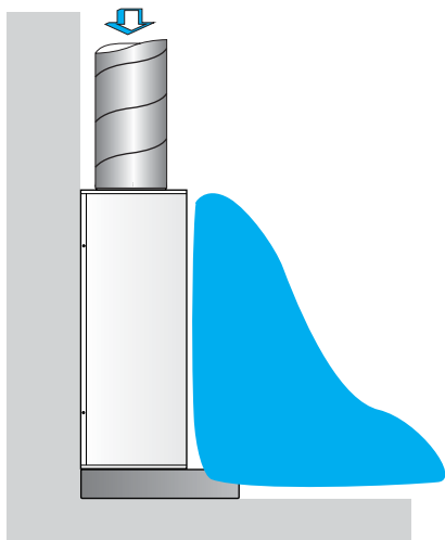
LSH anslutning ovanifrån, montage på vägg. Sockel (byggmaterial) mot golv som påkörningsskydd.
