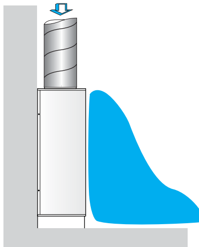
LSH anslutning ovanifrån, montage på vägg. Sockel SSH (tillbehör) mot golv.
